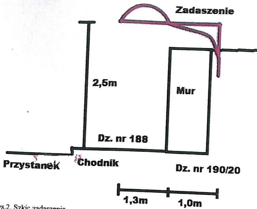
Rys.2. Szkic zadaszenia
