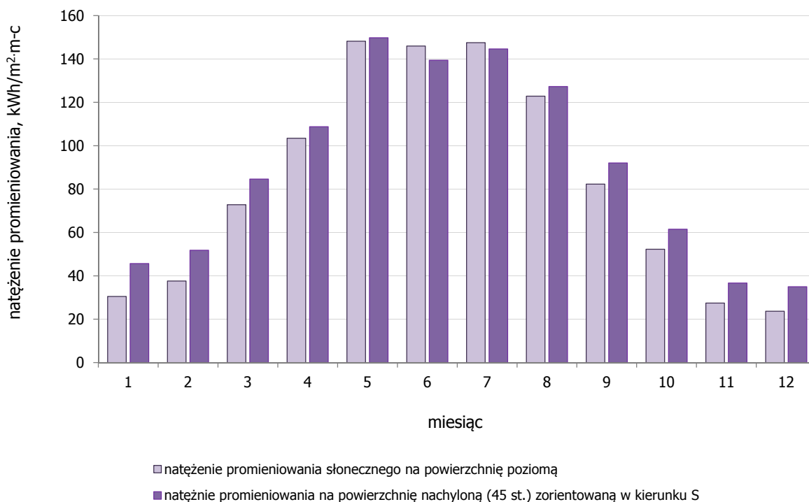
Rysunek 4.3 Energia promieniowania słonecznego na rozpatrywanym obszarze (natężenie promieniowania na powierzchnię poziomą oraz nachyloną pod kątem 45° dla danego miesiąca w ciągu roku)
